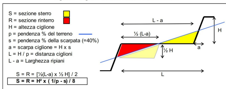
Figura 1 - Cigioni: calcolo sezioni sterri e rinterri
