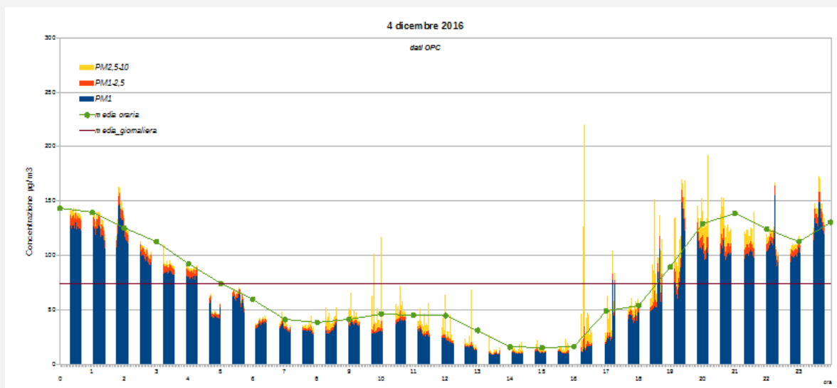
Figura 5 Andamenti dei vari contributi del PM (in blu frazione del PM1, in rosso frazione da PM1 a PM2,5 in giallo frazione tra PM2,5 e PM10). La curva verde riporta il valore della media oraria (riferita ai dati minuto precedenti), la retta marrone rappresenta la media giornaliera
