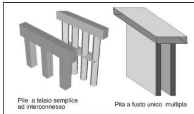
Figura 3 - Telaio diaframmato
