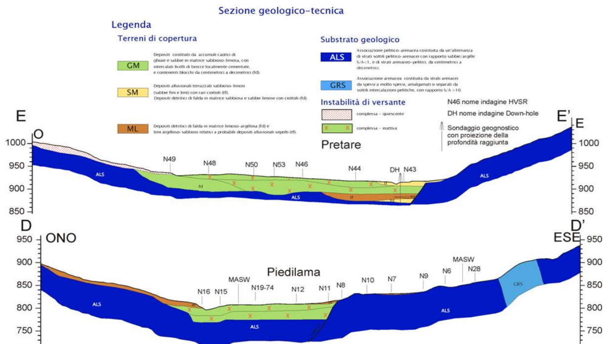
Figura 14 Sezioni Geologico-Tecniche dell'area di Pretare e Piedilama, realizzate nell'ambito degli Studi Microzonazione Sismica di III livello del Comune di Arquata del Tronto.
