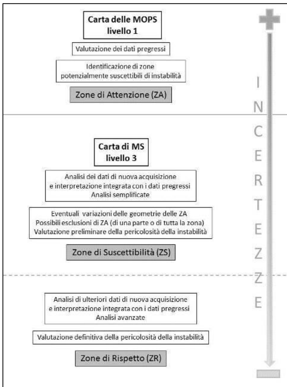
Figura 32 Schema che illustra i livelli di MS per la definizione delle zone suscettibili di instabilità. La raccolta dati e le analisi permettono di ridurre le incertezze dal livello 1 al livello 3.
