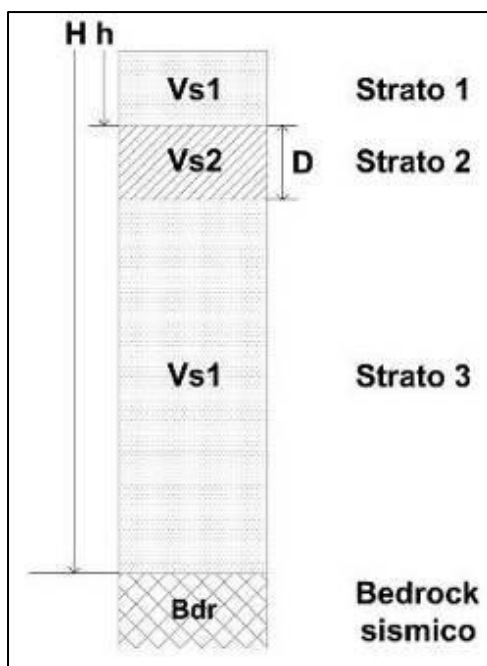
Figura 33 Esempio di colonna geologico-tecnica con inversione di velocità. Legenda simboli: H) profondità (m) rispetto al p.c. del tetto del bedrock sismico; h) profondità (m) rispetto al p.c. del tetto dello strato 2 (+soffice/+rigido); D) spessore (m) dello strato 2 (+soffice/+rigido); Vs1) velocità delle onde S (m/s) dello strato 1 e dello strato 3; Vs2) velocità delle onde S (m/s) dello strato 2 (+soffice/+rigido); Bdr) bedrock sismico. Il testo fa riferimento alla simbologia riportata in figura.
