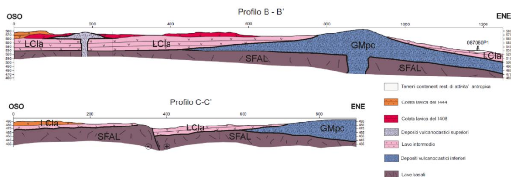
Figura 28 Stralcio di CGT_MS realizzata nell'ambito degli studi di MS di livello 1 del Comune di Trecastagni ( http://sit.protezionecivilesicilia.it/index.php?option=com_content&view=article&id=70&Itemid=187 , modificato).
