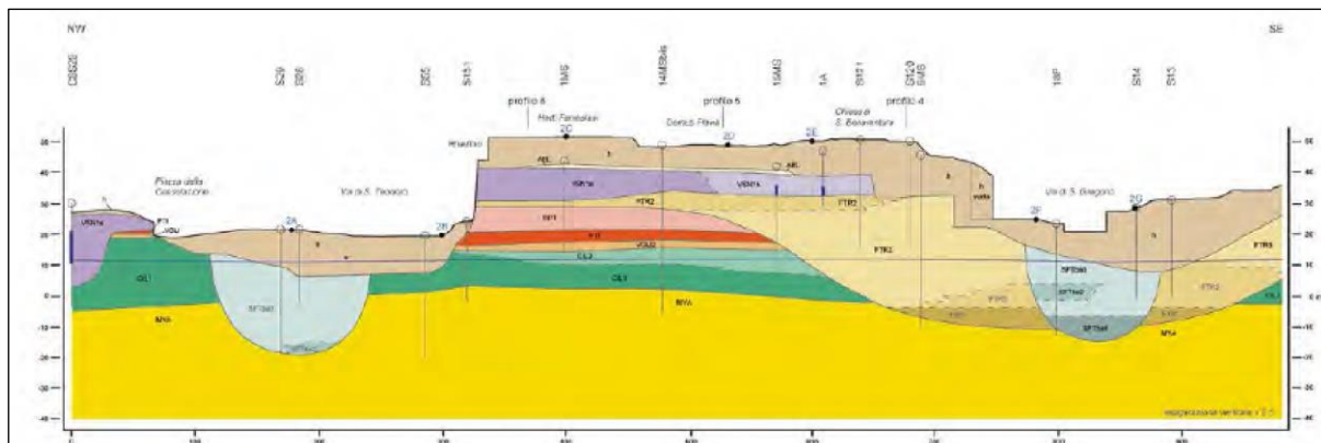
Figura 30 Sezione geologica tecnica attraverso l'Area Archeologica Centrale di Roma (M. Palatino). Si noti lo spessore della coltre antropica e l'estensione areale che copre completamente il substrato naturale e le morfologie sepolte (Moscatelli et al., 2012)
