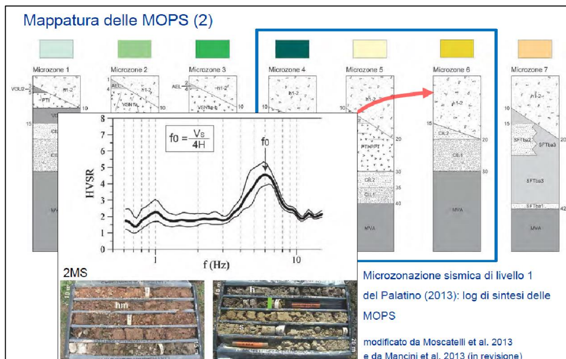
Figura 31 Colonne geologico tecniche del colle Palatino e risultati delle analisi di rumore ambientale. Alla frequenza di 6 Hz è presente una forte amplificazione dovuta allo spessore dello strato antropico e al contrasto di impedenza con le unità di copertura.
