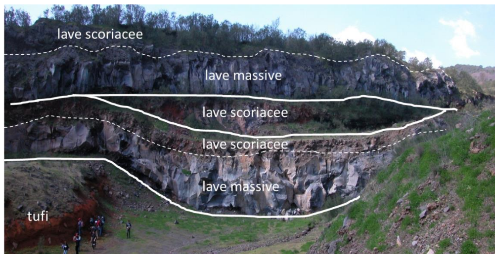
Figura 23 Fronte di cava nei pressi di Milo (fianco orientale dell'Etna) caratterizzato dalla presenza di tre distinti orizzonti lavici: quello più basso, costituito da una porzione inferiore litoide massiva e da una superiore scoriacea che mantella una paleovalle incisa sui tufi; la colata intermedia scoriacea che colma la paleovalle, mentre la colata superiore, anch'essa costituita da una porzione inferiore litoide e una superiore scoriacea, ricopre una topografia tabulare.
