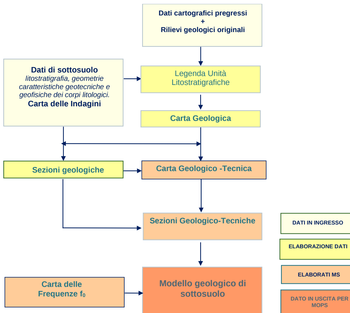
Figura 1 Percorso metodologico per produrre il modello geologico di sottosuolo. Da Castenetto (2013), modificato. Si noti come i dati del sottosuolo, contribuiscano sia alla stesura della CGT_MS che all'elaborazione delle sezioni geologiche tecniche. f_0 , frequenze fondamentali del terreno
