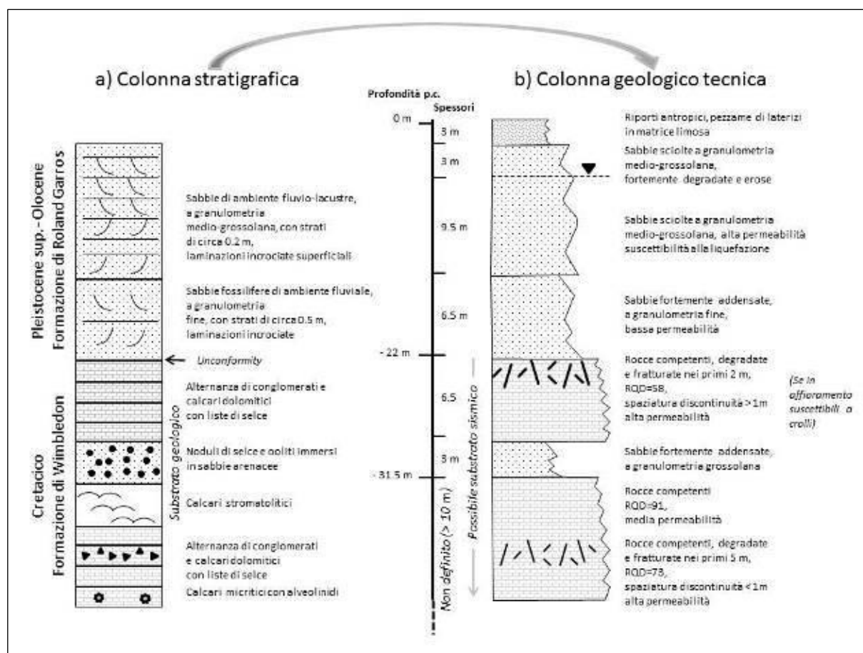
Figura 17 Esempio di colonna stratigrafica (a) e colonna geologico-tecnica (b) a confronto.
