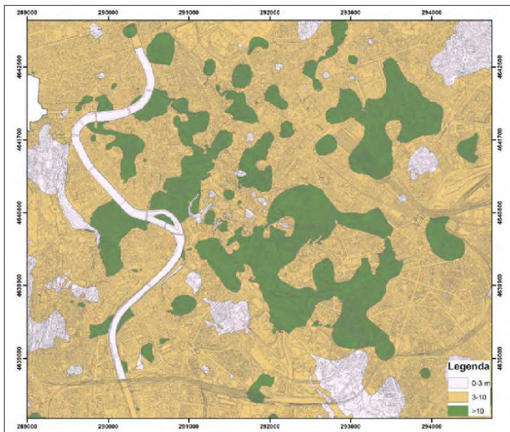
Figura 29 Cartografia dello strato antropico del centro storico di Roma. Da (Moscatelli et al., 2013).
