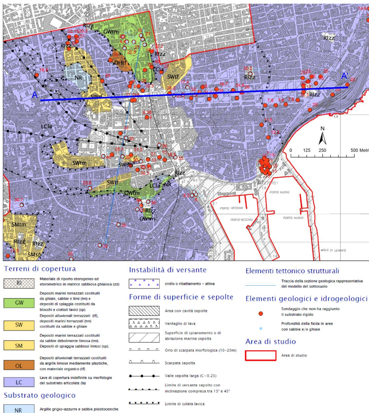
Figura 27 Stralcio di CGT_MS realizzata nell'ambito degli studi di MS di livello 1 dell'area urbana di Catania ( http://sit.protezionecivilesicilia.it/index.php?option=com_content&view=article&id=70&Itemid=187 , modificato).
