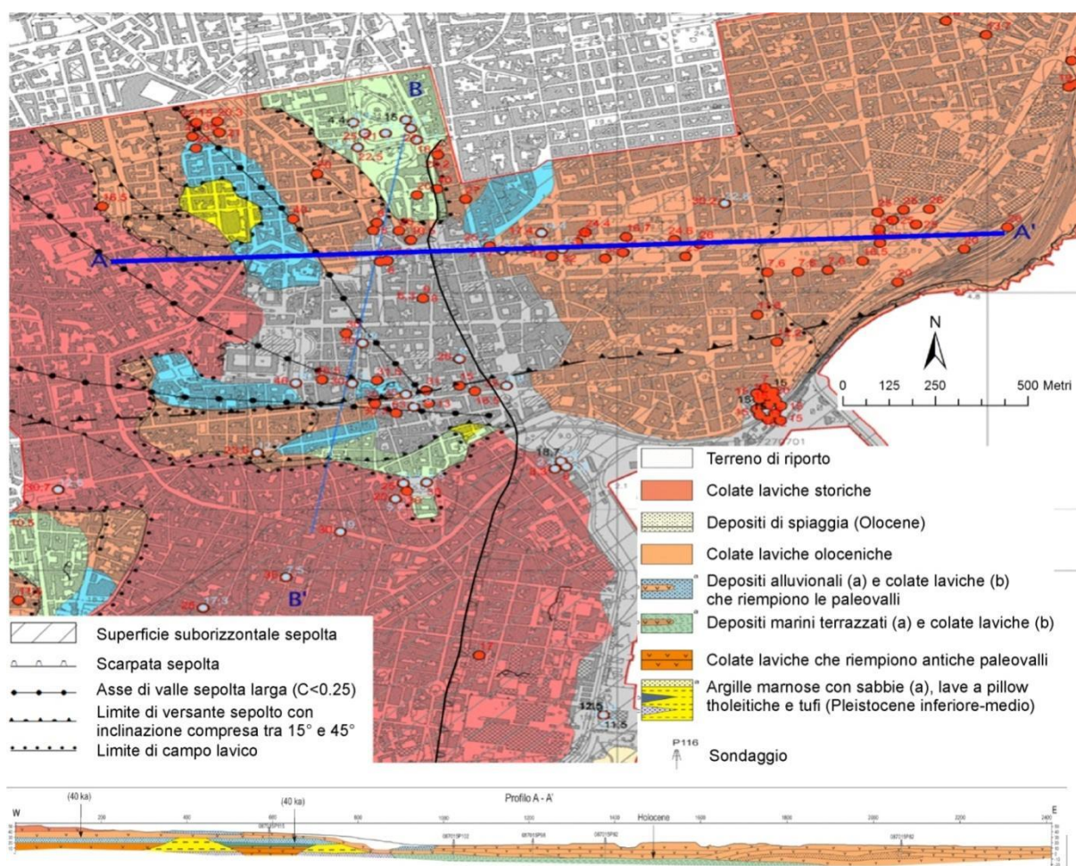
Figura 26 Stralcio di Carta Geologica(CG) realizzata nell'ambito degli studi di MS di livello 1 dell'area urbana di Catania e sezione geologica A-A' ( http://sit.protezionecivilesicilia.it/index.php?option=com_content&view=article&id=70&Itemid=187 , modificato).
