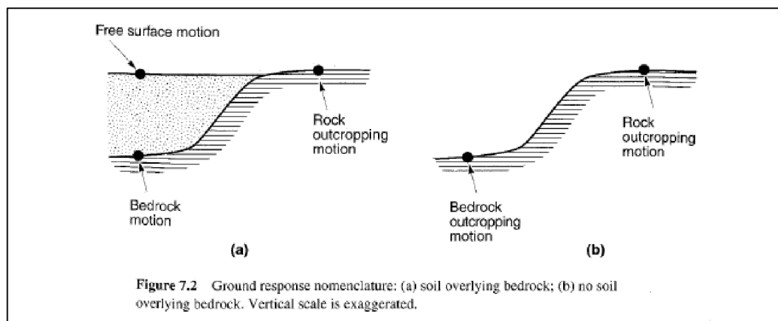
Figura 19 Esempi di substrato. La figura è ripresa da (Kramer, 1996). Interessante è la nomenclatura adottata dall'Autore; free surface: punto sommitale della successione dei terreni soffici; bedrock: substrato sismico al di sotto della successione dei terreni soffici; rock outcropping: roccia affiorante; bedrock outcropping: substrato sismico affiorante (non sovrastato da terreni soffici).
