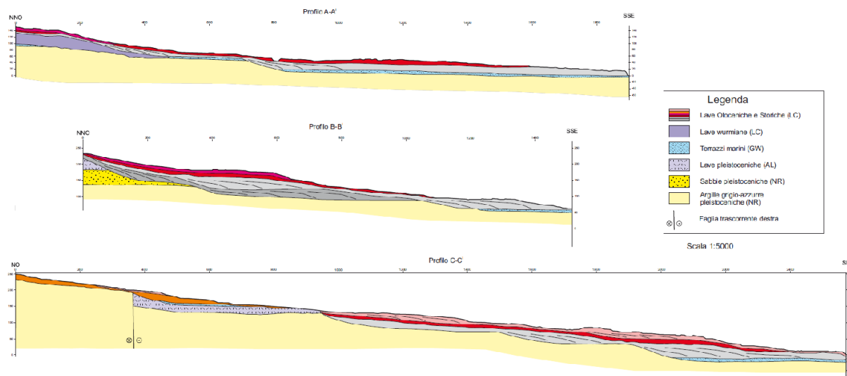
Figura 25 Sezioni geologiche realizzate nell'ambito degli studi di MS di livello 1 del Comune di Aci Castello ( http://sit.protezionecivilesicilia.it/index.php?option=com_content&view=article&id=62&Itemid=185 )
