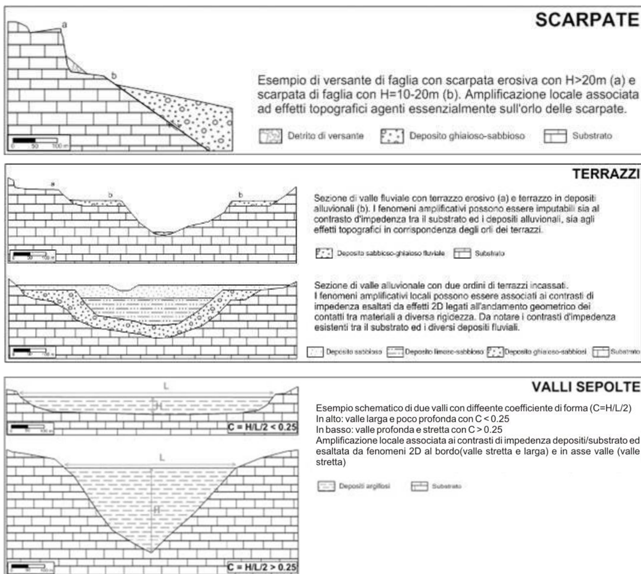
Figura 22 Esempi semplificati di assetti morfologici e geologici che possono condizionare la risposta sismica in superficie.
