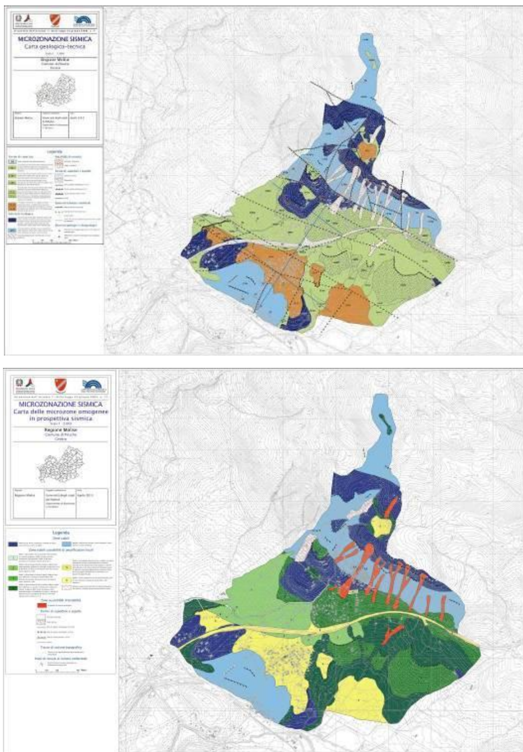
Figura 18 a) Carta geologico-tecnica con affioramenti di substrato geologico; b) Carta delle MOPS con zone stabili (affioramenti del substrato geologico).
