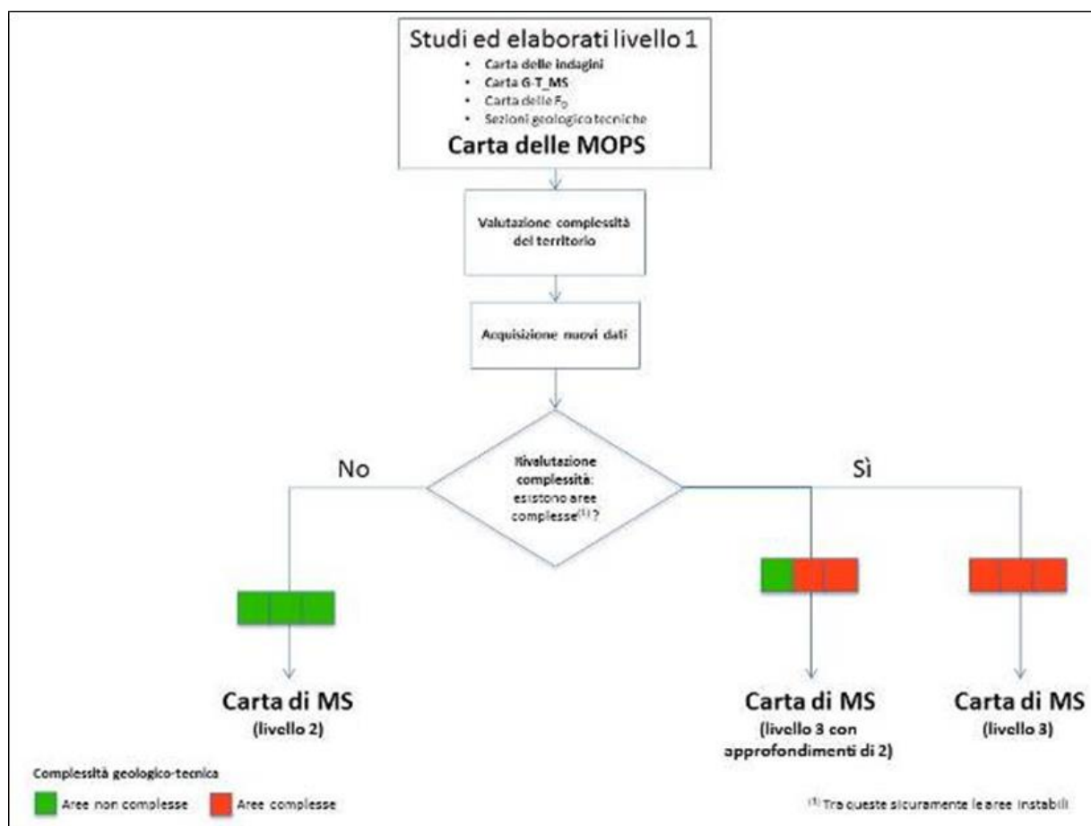
Figura 4 Percorso metodologico per l'elaborazione delle carte di MS e utilizzo della CGT_MS e delle sezioni geologico tecniche.
