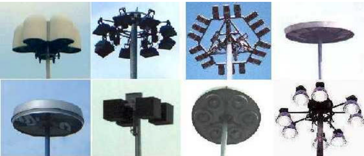
Figura 18 - Esempi di torri faro perfettamente schermate, in questo caso la luce è diretta esclusivamente verso il basso, dove realmente serve.
