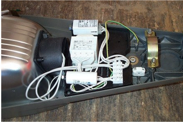
Figura 25 - Elementi di cablaggio elettrico.
