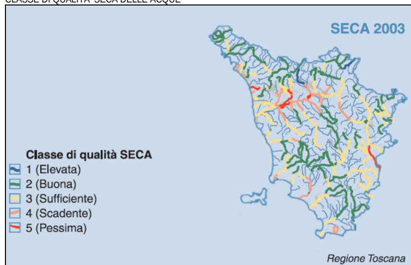
Figura 3.29 CLASSE DI QUALITÀ SECA DELLE ACQUE
