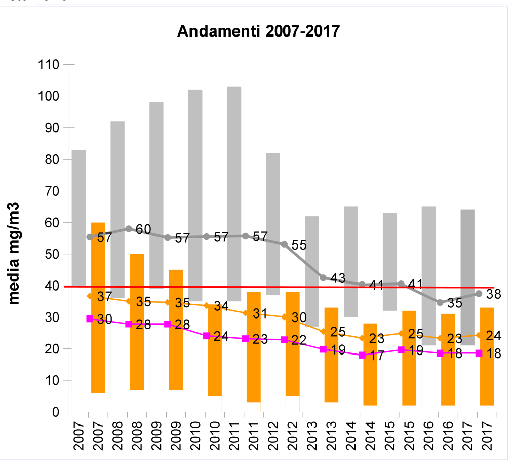
Grafico 4.3.6. NO 2 – Andamenti della concentrazione media annuale dal 2007 al 2017 per tipologia di stazione.
