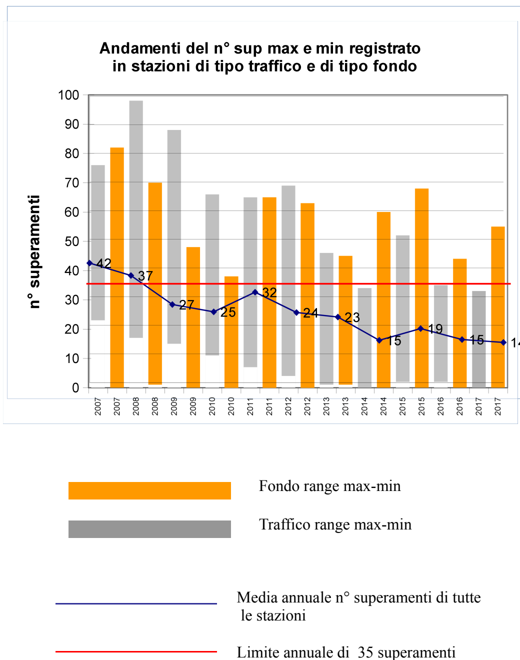
Grafico 4.1.11 PM10 – Andamenti del numero massimo e minimo di superamenti dal 2007 al 2017 per tipologia di stazione.
