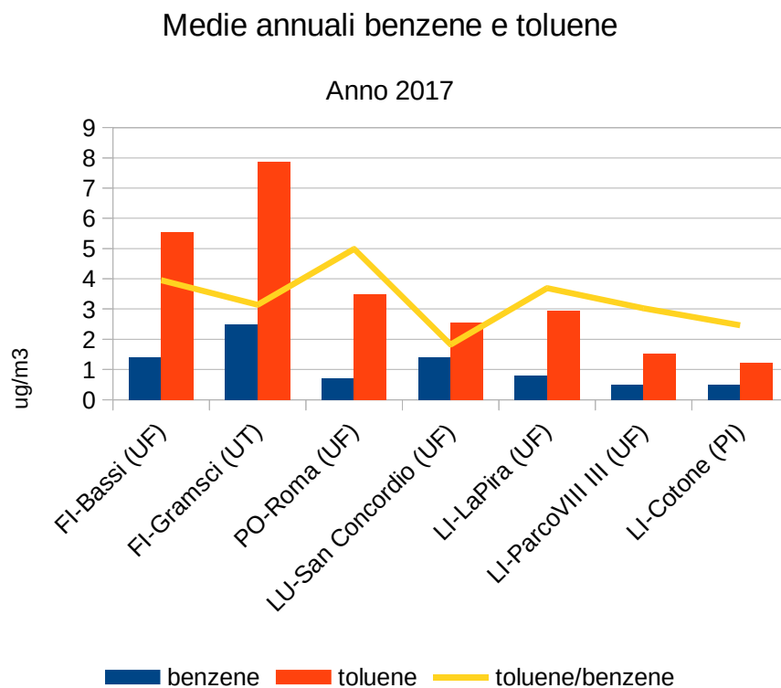
Grafico 4.8.5. Valori medi annuali 2017 di benzene e toluene e loro rapporto.
