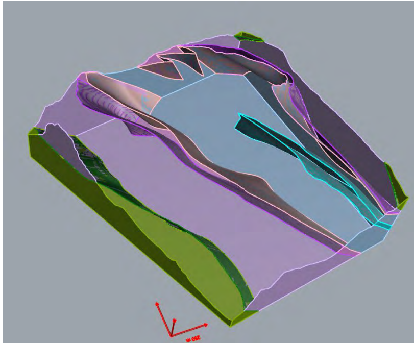
Figura 31 - Modello tridimensionale del Monte Corchia in cui sono state inserite quattro superfici laterali verticali ed una superfici di base piana inclinata.
