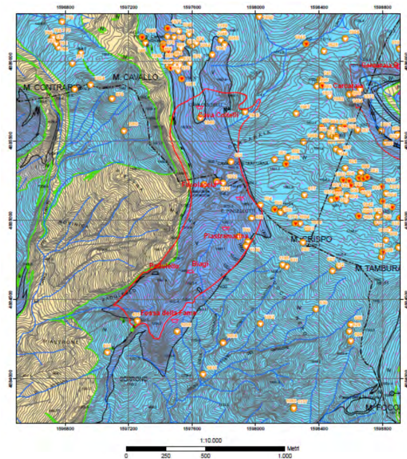
Figura 21 - Carta Idrogeologica relativa all'area contigua del Monte Cavallo (Comune di Massa e di Minucciano).
