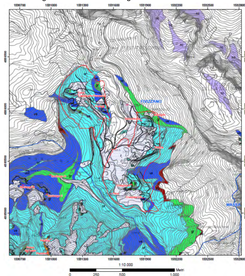
Figura 22 - Carta delle varietà merceologiche delle aree contigue Monte Sagro Morluno e Monte Borla (Comune di Fivizzano)
