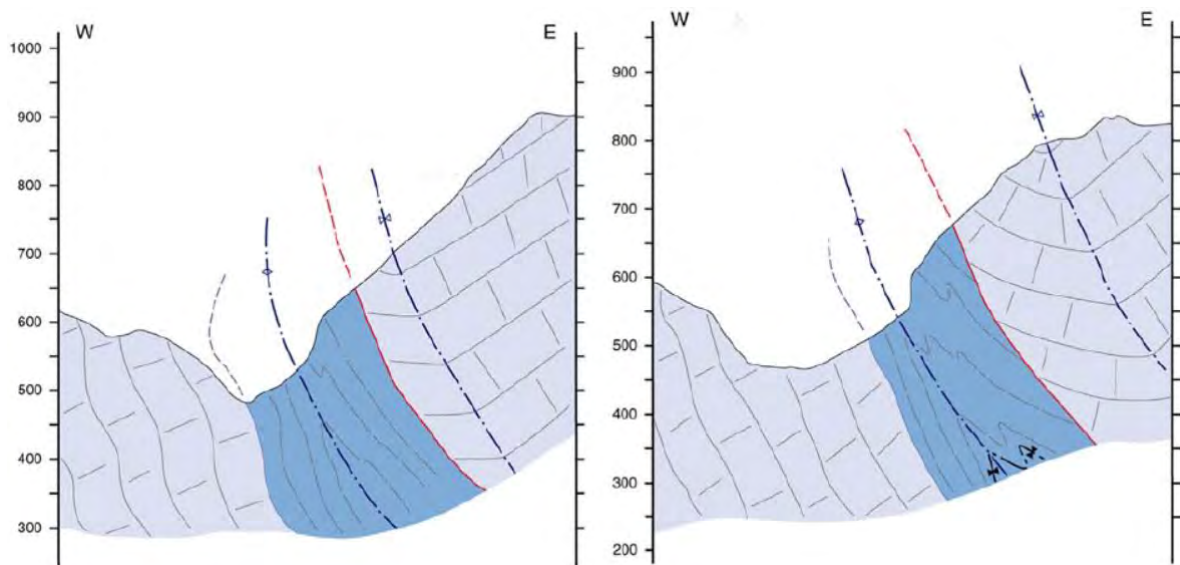
Figura 24 - Sezioni utilizzate per la ricostruzione geologica tridimensionale del giacimento di marmo relativo all'area contigua Fondone Cerignano nel Comune di Massa. (da Vanneschi et alii., 2014).
