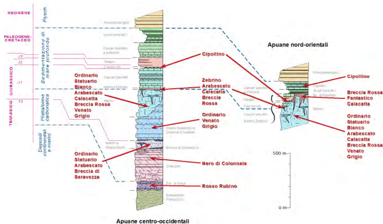
Figura 5 - Le varietà merceologiche di marmi (indicate in rosso) nella successione metamorfica delle Alpi Apuane. Basamento Paleozoico: filladi, porfiroidi, scisti porfirici, dolomie, filladi grafitiche e calcescisti (?Cambriano - ?Devoniano); Formazione di Vinca: filladi, quarziti e metaconglomerati alternati a dolomie, marmi, marmi dolomitici, e metabrecce poligeniche (Carnico - ?Norico); Grezzoni: dolomie, dolomie brecciate e marmi neri alternati a dolomie (Norico); Marmi a Megalodonti e Breccie di Seravezza: marmi, metabrecce poligeniche e scisti a cloritoide; Marmi Dolomitici: marmi, marmi dolomitici e dolomie (Lias Inf); Marmi: marmi e metabrecce monogeniche (Lias Inf); Marmo Zerbino: marmi, metabrecce e calcescisti (Lias Inf - ?Medio); Formazione di Arnetola: metabrecce poligeniche (Lias inf - ?Cretaceo); Calcarei Selciferi: metacalcilutiti con liste e noduli di selce (Lias Medio - Sup); Calcescisti: calcescisti e filladi carbonatiche (Lias Sup); Diaspri: metaradiolariti e filladi quarzitiche (Malm); Calcarei Selciferi a Entrochi: metacalcilutiti con liste e noduli di selce bianche
