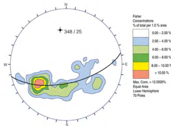
Figura 23 - Analisi statistica relativa alla dispersione della scistosità principale finalizzata all'individuazione dell'asse medio della struttura dell'antiforme del Monte Rasori presso la cava Romana (area contigua Fondone Cerignano) (da Vanneschi et alii., 2014).
