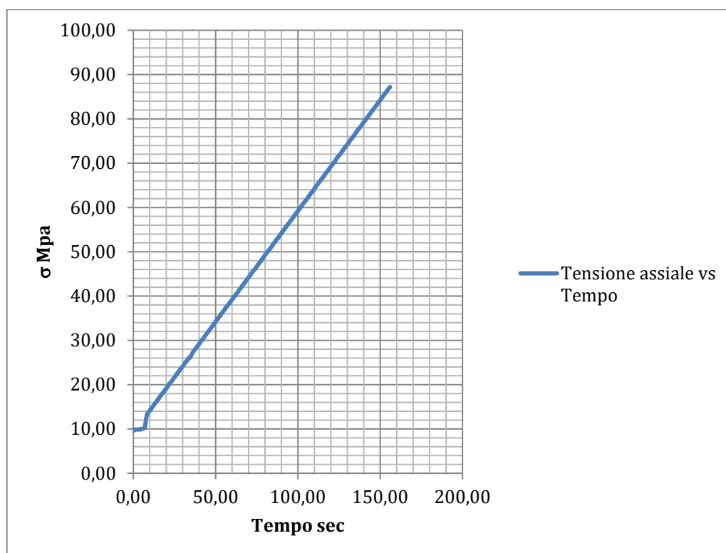
Figura 11 - Andamento della tensione assiale espressa in MPa, rispetto al tempo di prova in secondi.
