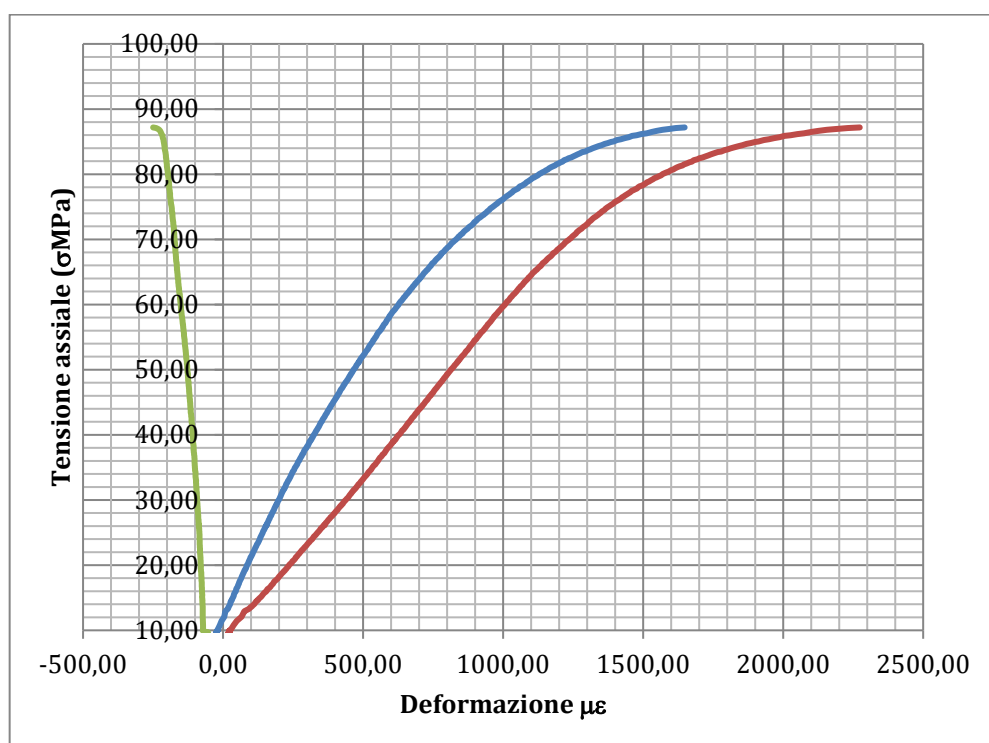
Figura 12 - Andamento della tensione assiale (MPa) Vs deformazione assiale (curva azzurra e rossa) e della deformazione diametrale (curva verde) (microepsilon).
