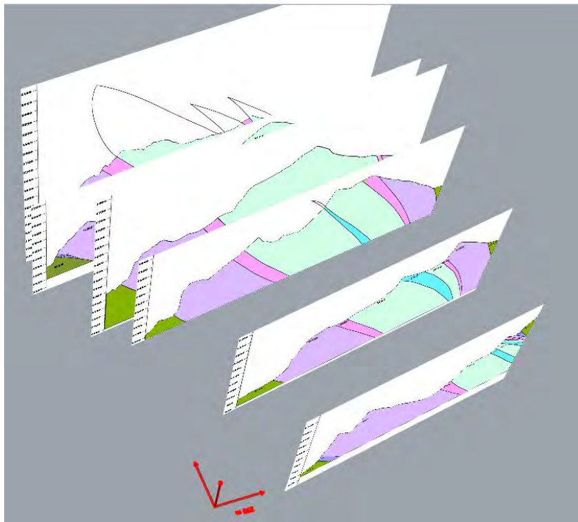
Figura 28 - Sezioni geologiche seriate utilizzate per la realizzazione del modello tridimensionale della geologia del Monte Corchia. La formazione marmifera è indicata di colore celeste chiaro.
