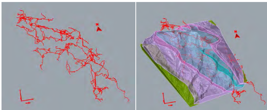
Figura 35 - A sinistra complesso carsico del Monte Corchia rappresentato in tre dimensioni. A destra modello geologico tridimensionale del Monte Corchia comprensivo dello sviluppo sotterraneo del sistema carsico. In azzurro è rappresentata la formazione marmifera.
