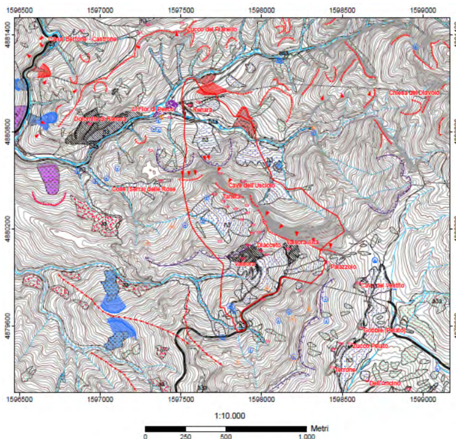
Figura 19 - Allegato 3 Esempio di Carta Geomorfologica relativa all'area contigua Valsora Giacceto nel Comune di Massa.
