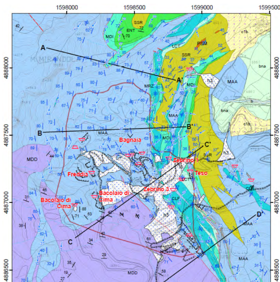
Figura 20 - Stralcio dell'Allegato 4: Carta geologica relativa all'area contigua della Carcaraia nel Comune di Minucciano.
