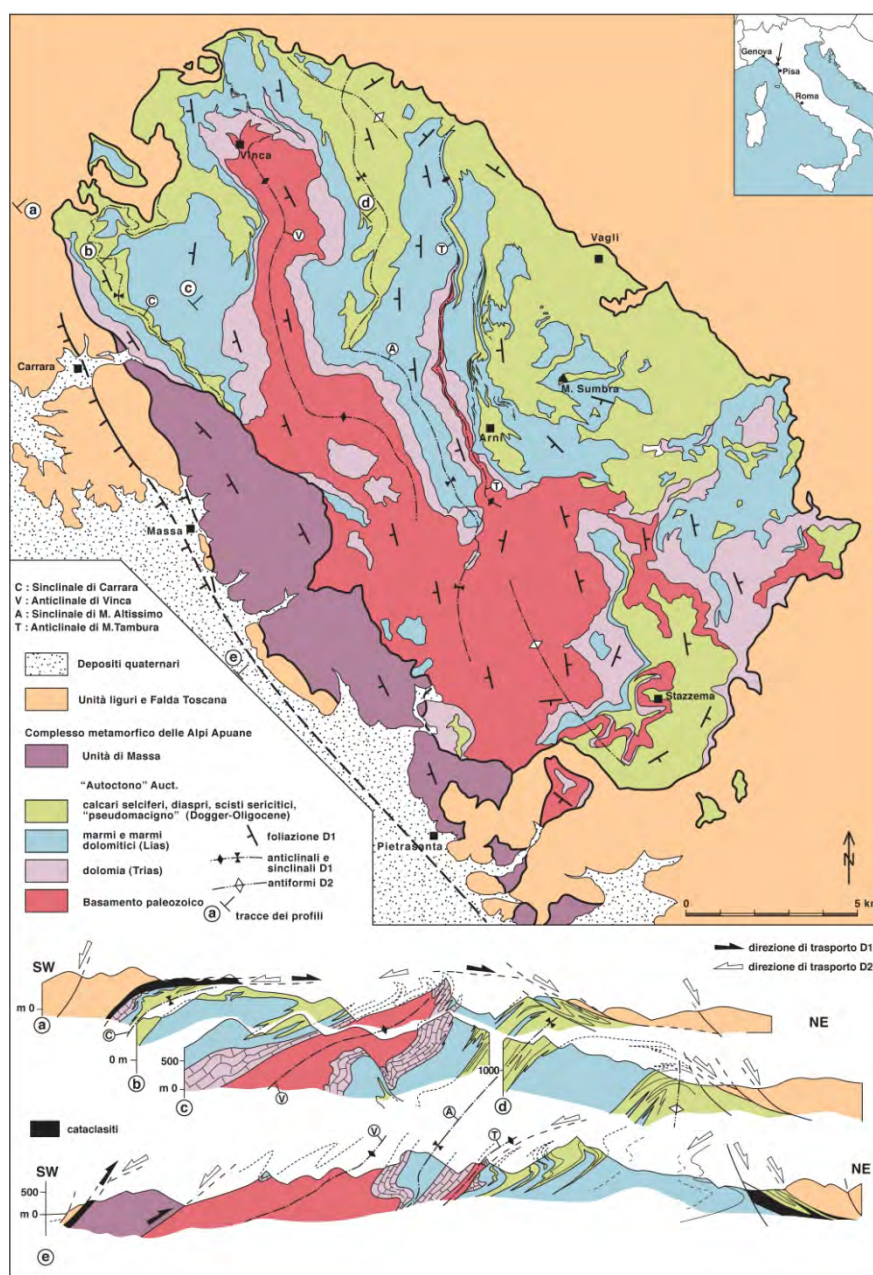
Figura 3 - Schema tettonico delle Alpi Apuane.
