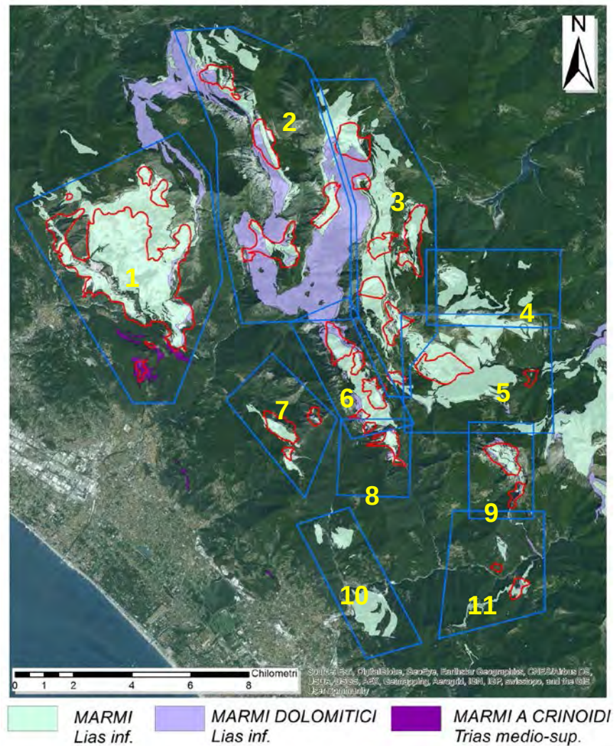
Figura 14 - In celeste sono rappresentati gli affioramenti di marmo dell'Unità dell'"Autoctono" Auct., in viola i marmi triassici dell'Unità di Massa ed in viola chiaro i Marmi dolomitici. Sono numerati gli undici domini strutturali omogenei: 1: Dominio di Carrara ; 2: Dominio Orto di Donna ; 3: Dominio Monte Tambura Monte Sella; 4: Dominio Boana; 5: Dominio Turrile Secca; 6: Dominio Monte Altissimo; 7: Dominio Madielle; 8: Dominio Crevaiole; 9: Dominio Monte Corchia; 10: Dominio Trambiserra Monte Costa; 11: Dominio Stazzemese. In rosso sono indicate le aree contigue di cava così come perimetrate dal Parco delle Alpi Apuane (L.R. n. 65/1997) (ad esclusione di quelle relative al Bacino 21 del PIT nell'area di affioramento della Formazione dello Pseudomacigno).
