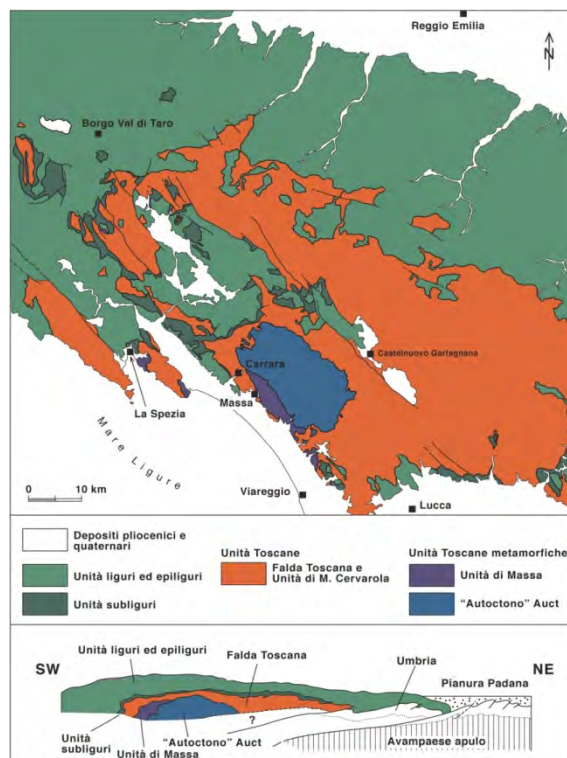
Figura 2 - Schema delle unità tettoniche dell'Appennino Settentrionale.
