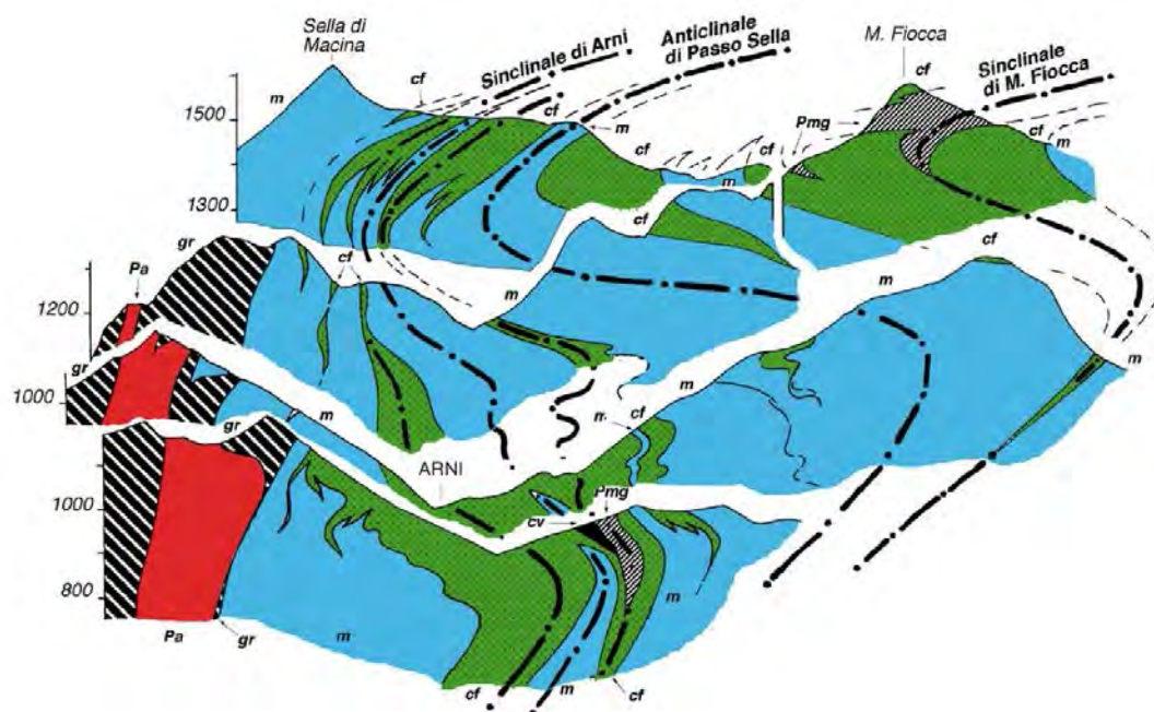
Figura 4 - Sezione composita della valle di Arni orientata in direzione Ovest-Est. Chiave di lettura delle sigle: Pa Basamento paleozoico; gr Grezzoni; m Marmo; cf Metacalcari selciferi, Metacalcari selciferi ad Entrochi, Metaradiolariti; Pmg Pseudomacigno.
