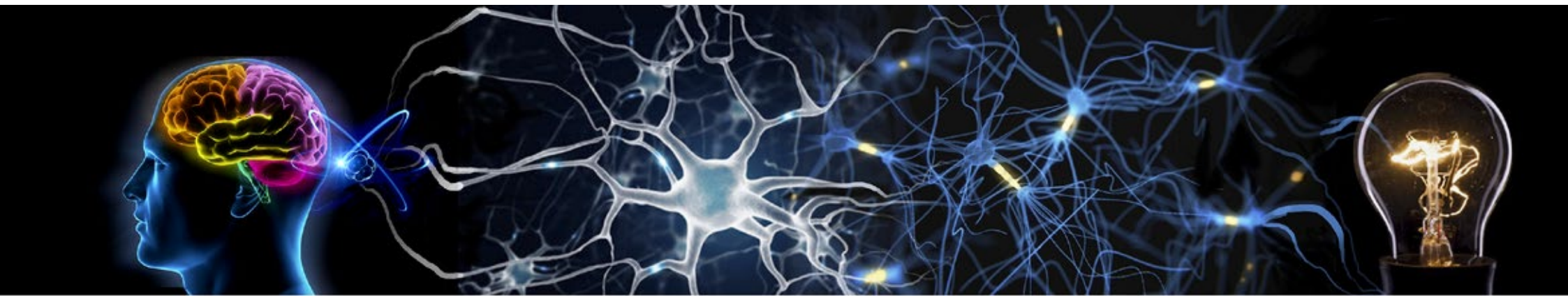
Migrazione degli elettroni da una molecola all'altra.
