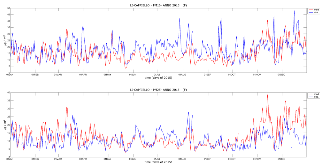
Figura 19. Serie storiche di confronto tra i dati da stazione (blu) e da modello (rosse) relative alla stazione di LI-Cappiello.
