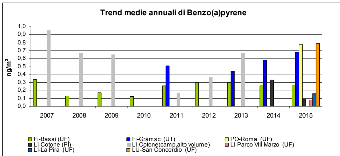
Grafico 5.1.2. Benzo(a)pirene. Medie annuali _ Andamenti 2007-2015
