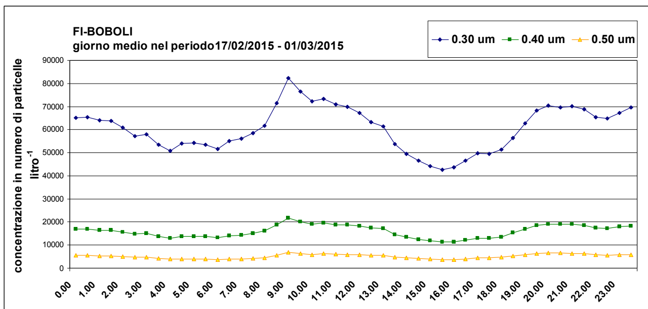
Figura 7. FI-BOBOLI Giorno medio 17/02/2015 - 01/03/2015
