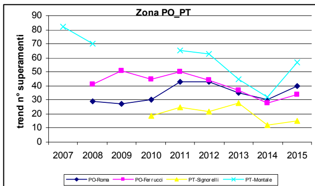
Grafico 4.1.4. PM10 - n° superamenti valore giornaliero 50 \mu\text{g}/\text{m}^3 - Andamenti 2007-2015 per zone.
