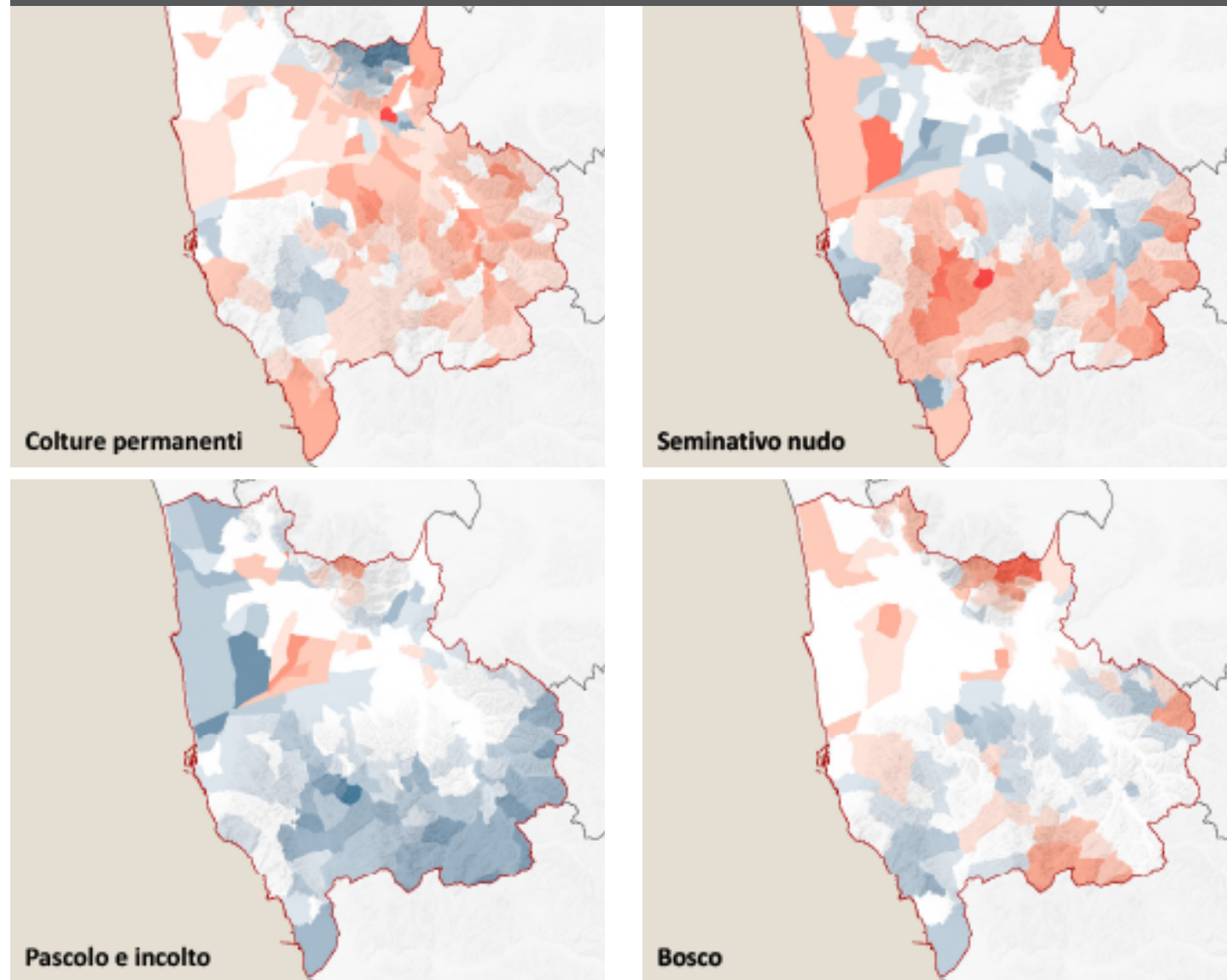
Variazioni dell'uso del suolo fra 1830 e 1960
