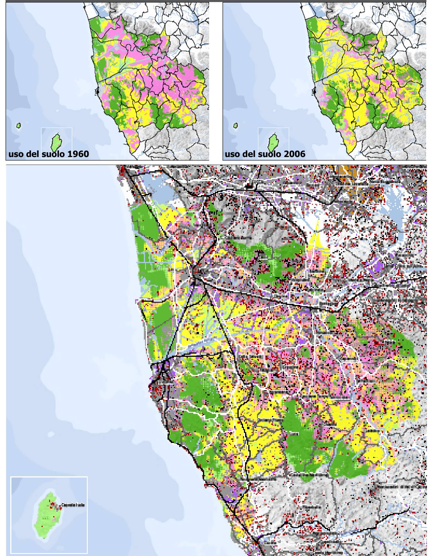
Variazioni dell'uso del suolo fra 1960 e 2006
