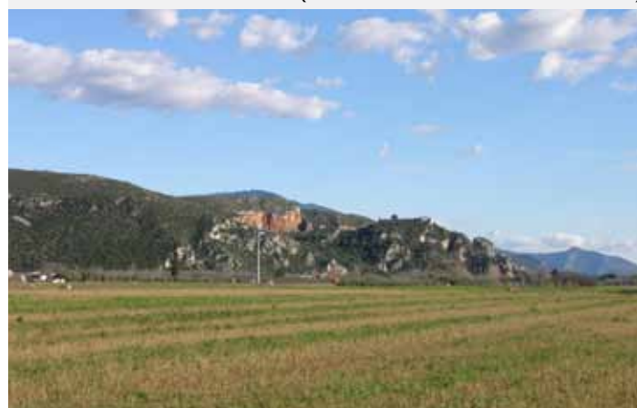
Rilievi calcarei nei pressi di Vecchiano (Foto B. Baldi)
