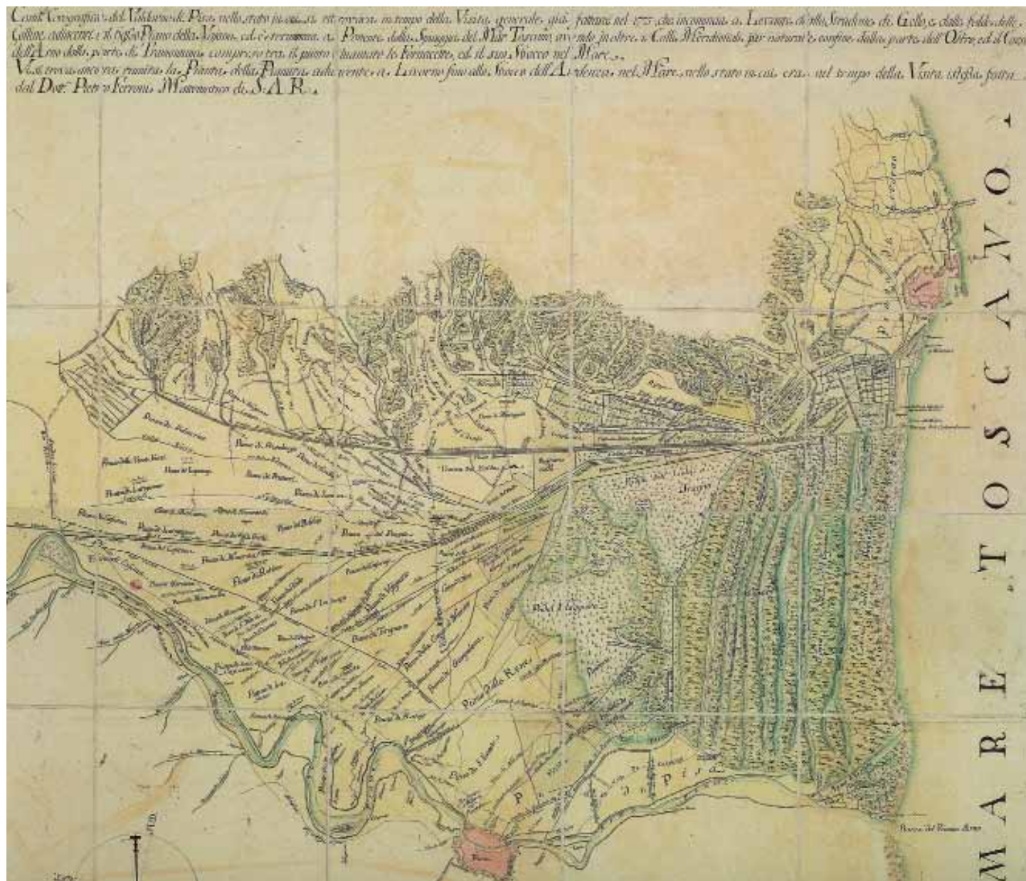
La Pianura Pisana nel 1774 (Stefano Diletti con la direzione di Pietro Ferroni, Archivio Nazionale di Praga)
