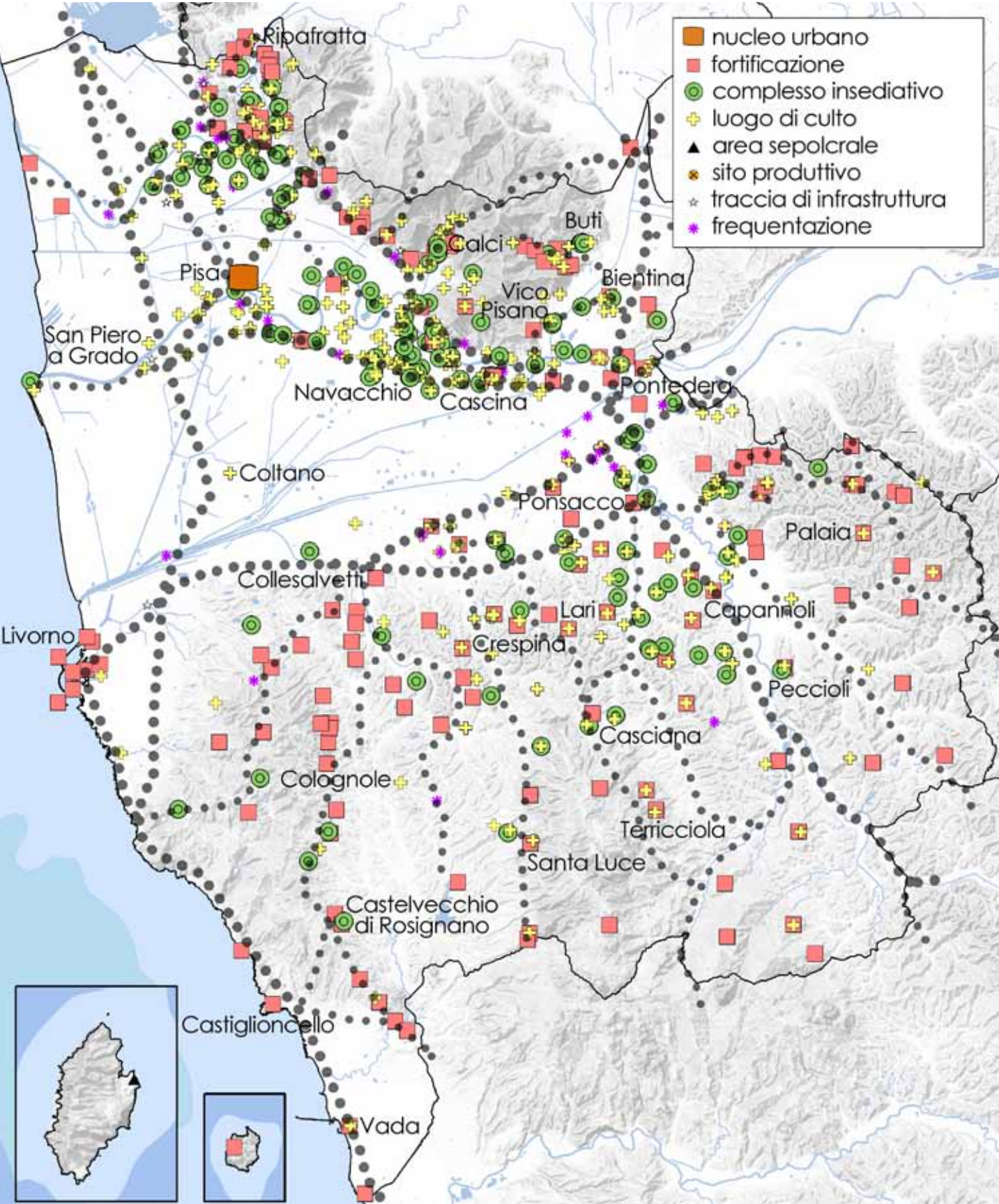
Rappresentazione della rete insediativa di periodo medievale sulla base dell'informazione archeologica edita, con ipotesi delle direttrici di transito e comunicazione (tracciati restituiti con pallini neri: più grandi per la viabilità primaria, più piccoli per quella secondaria) e ricostruzione della linea di costa (tratteggio e campitura azzurra). Scala 1: 260.000.
