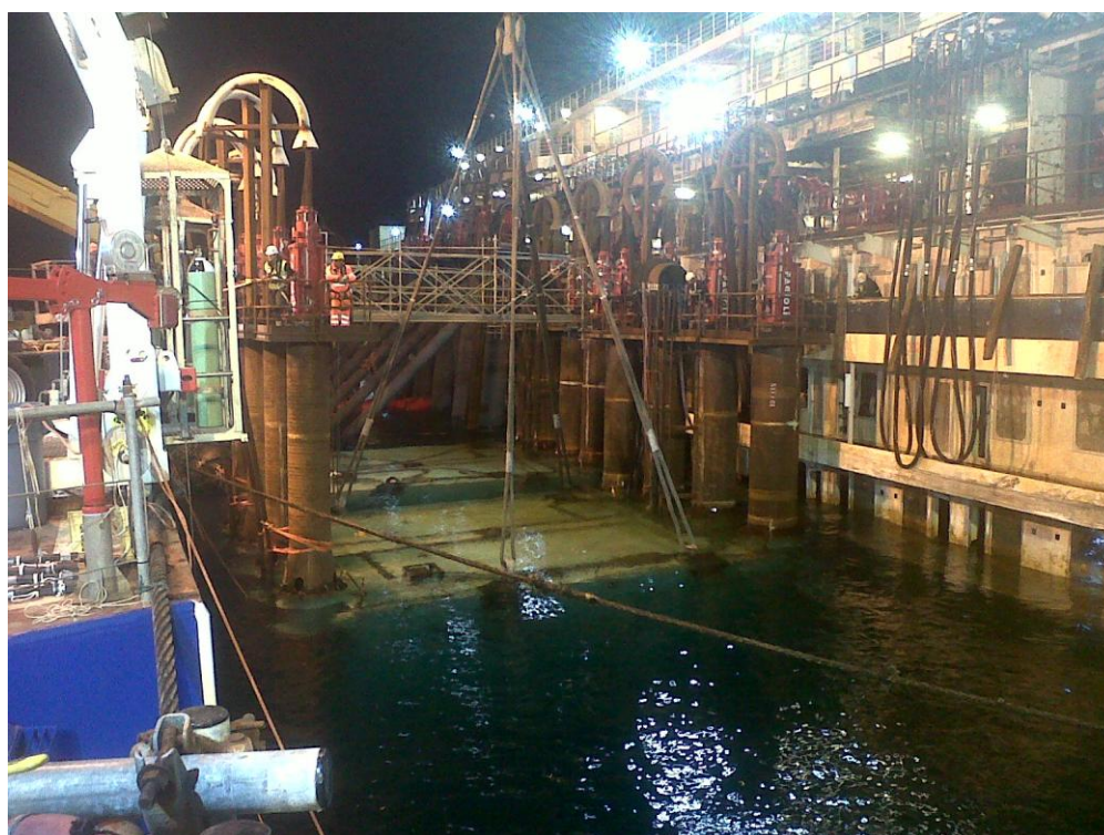
Sopra: Operazioni di taglio dei tubolari della piattaforma 2 Sotto: Installazione cassone S11
